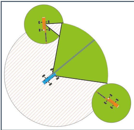
Figuur 1. bovenaanzicht meerdere kranen in elkaars draaibereik.
